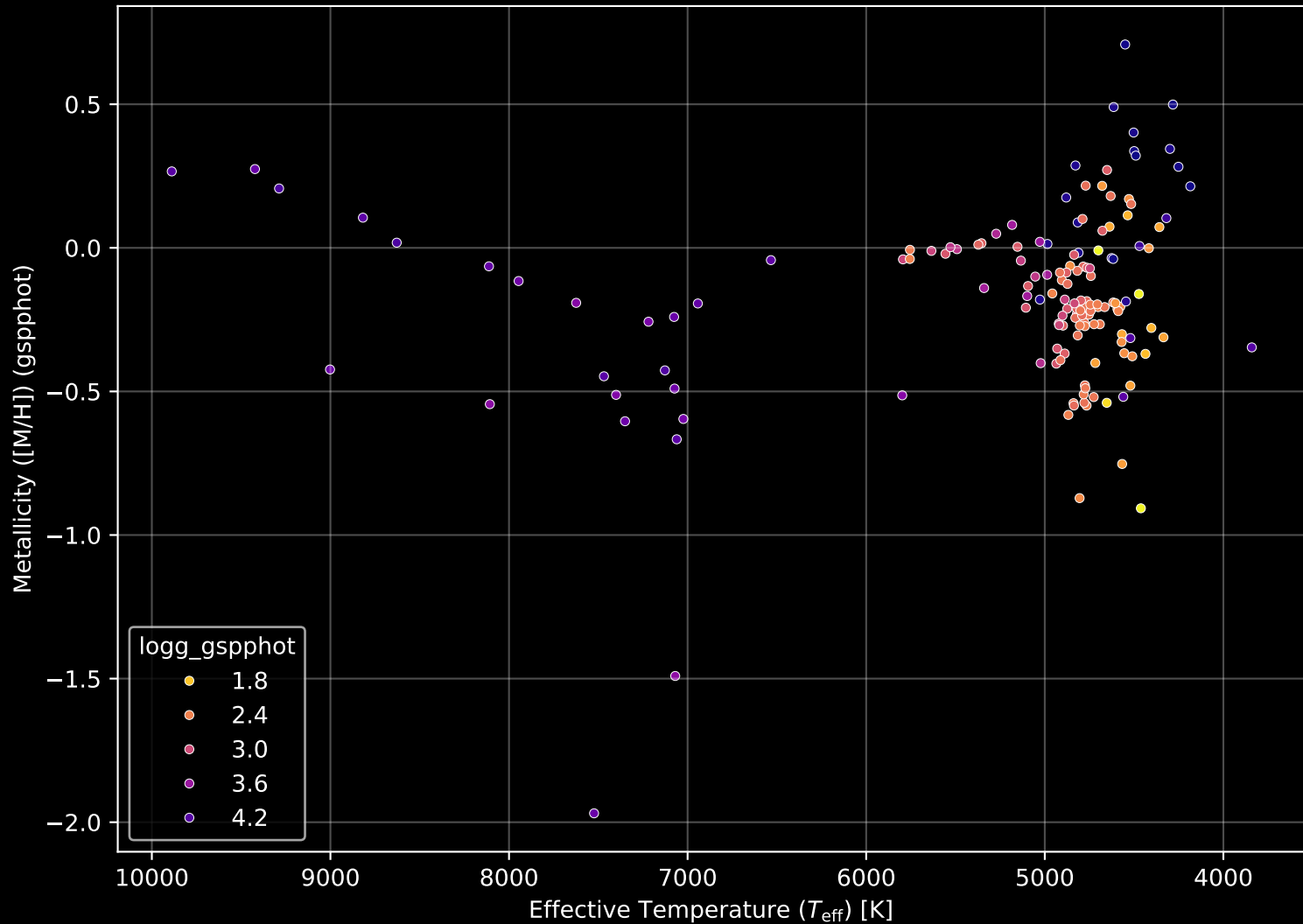
APOGEE DR17 Field: [240+18] Stellar Population Parameters (n= 154)
